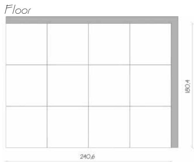
Floor Amarcord Sabbia Cerato RET 60x60 cm
