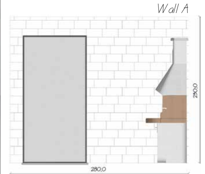
Wall covering Pietre di Fiume Multicolor 13x25 cm
